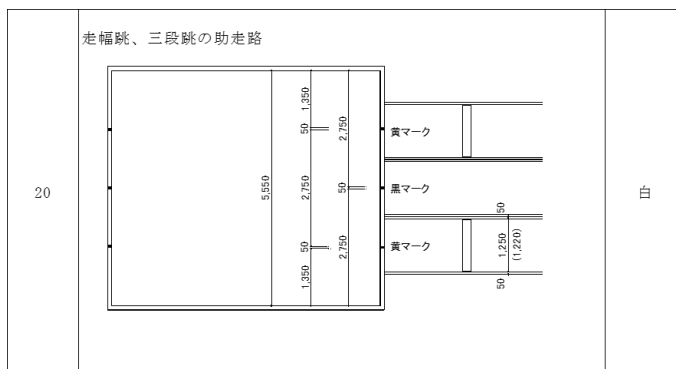
別表1 全天候舗装用レーンマーキング色分け標準表
