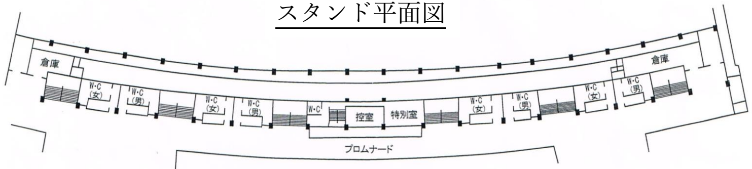
2階平面図
